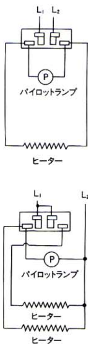
■結線図
