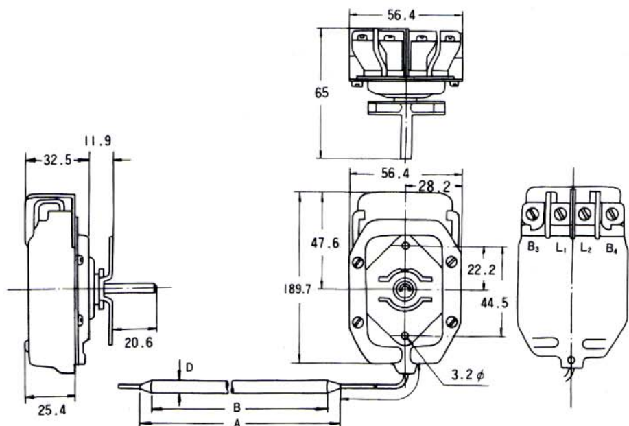
■寸法図
