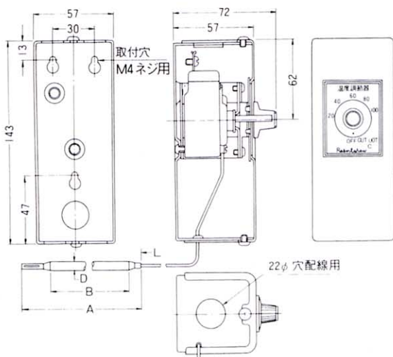
■EAC寸法図
